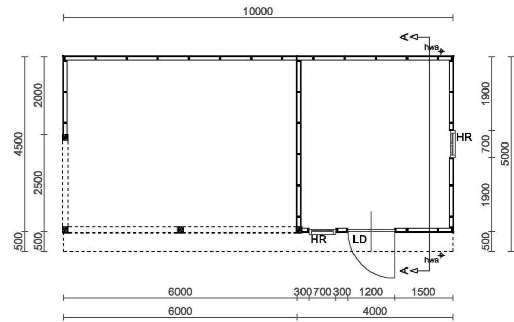
plattegrond
